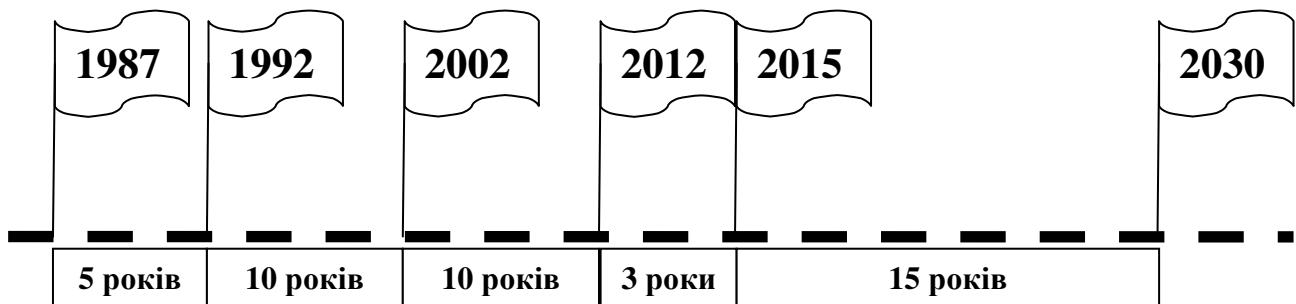
Рис. 2. Періодичність перегляду глобальних цілей сталого розвитку на рівні ООН з 1987 р.
