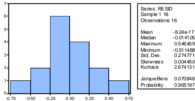
Рис. 1. Описова статистика залишків
